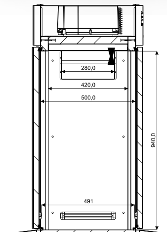
RIC1PTH Pasante/Pass-thru/Traversante
